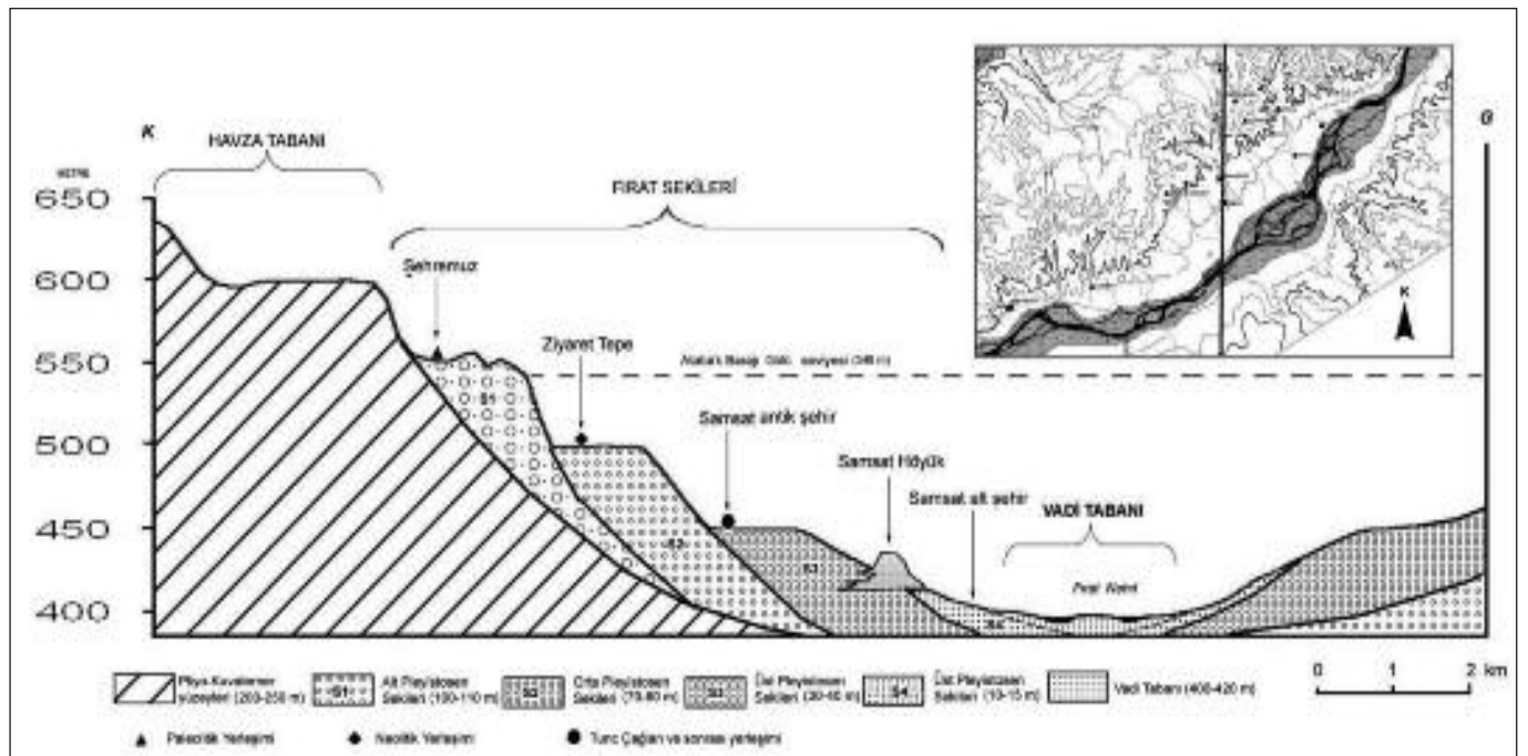
■ Şekil 3. Adıyaman'ın güneydoğusundaki Fırat vadisinde bazı tarihi yerleşme ve buluntu yerlerinin dağılımını gösteren topografik-jeomorfolojik kesit (Karadoğan ve Tonbul, 2007).
