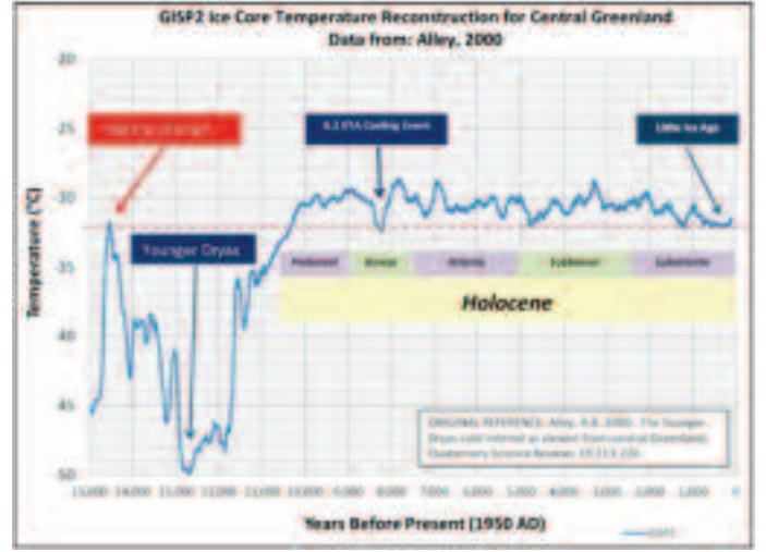
■ Şekil 2. Greenland'da son 15 bin yıldaki sıcaklık anomalileri, Bolling-Allerod ve Younger Dryas.
